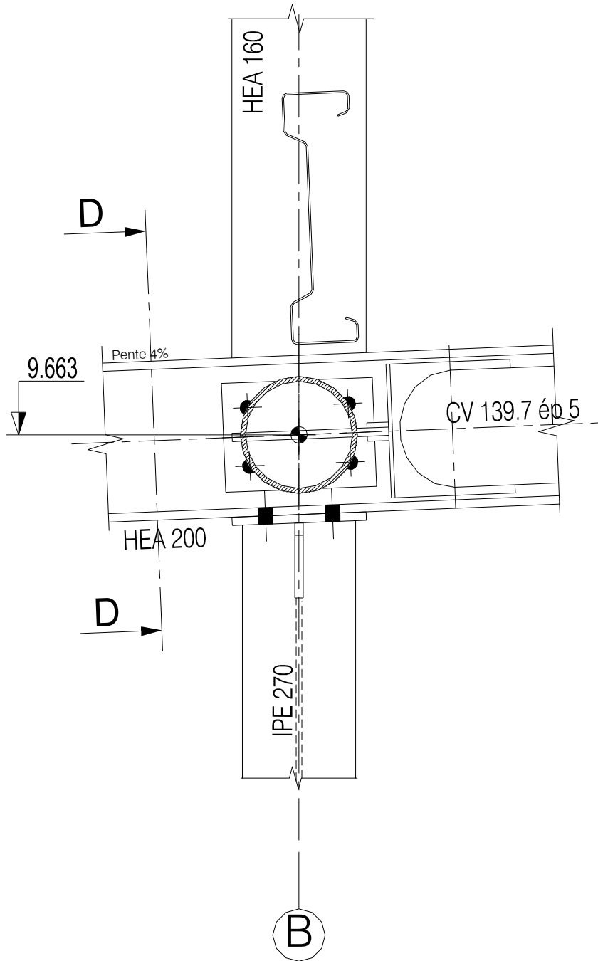
vue en élévation
